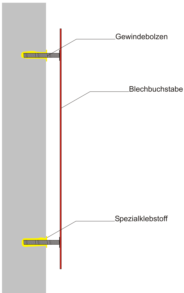
Befestigung durch Einkleben
