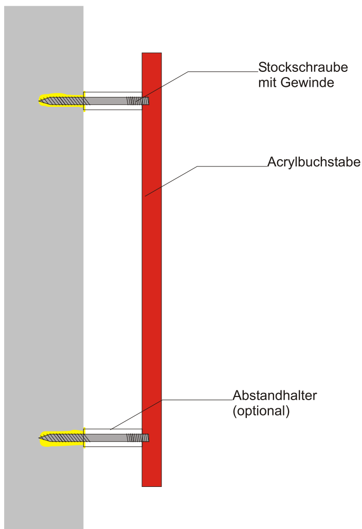
Befestigung durch Einkleben
